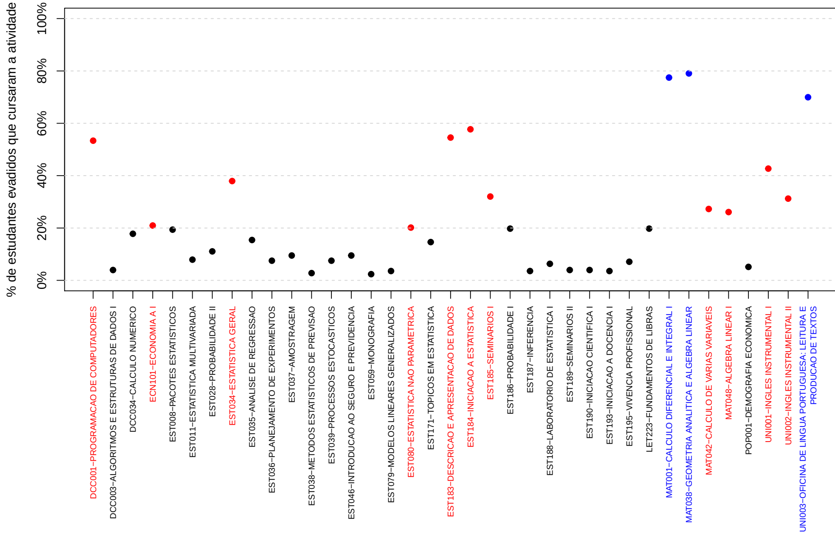
Figura 13: Principais atividades acadêmicas curriculares cursadas pelos estudantes que evadiram do curso de Estatística, modalidade Bacharelado.
