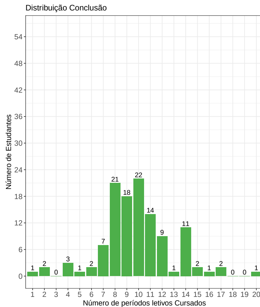
Figura 10: Número de períodos letivos cursados de acordo com a situação do estudante no curso de Estatística, modalidade Bacharelado, no período de 2010/1 a 2020/2.
