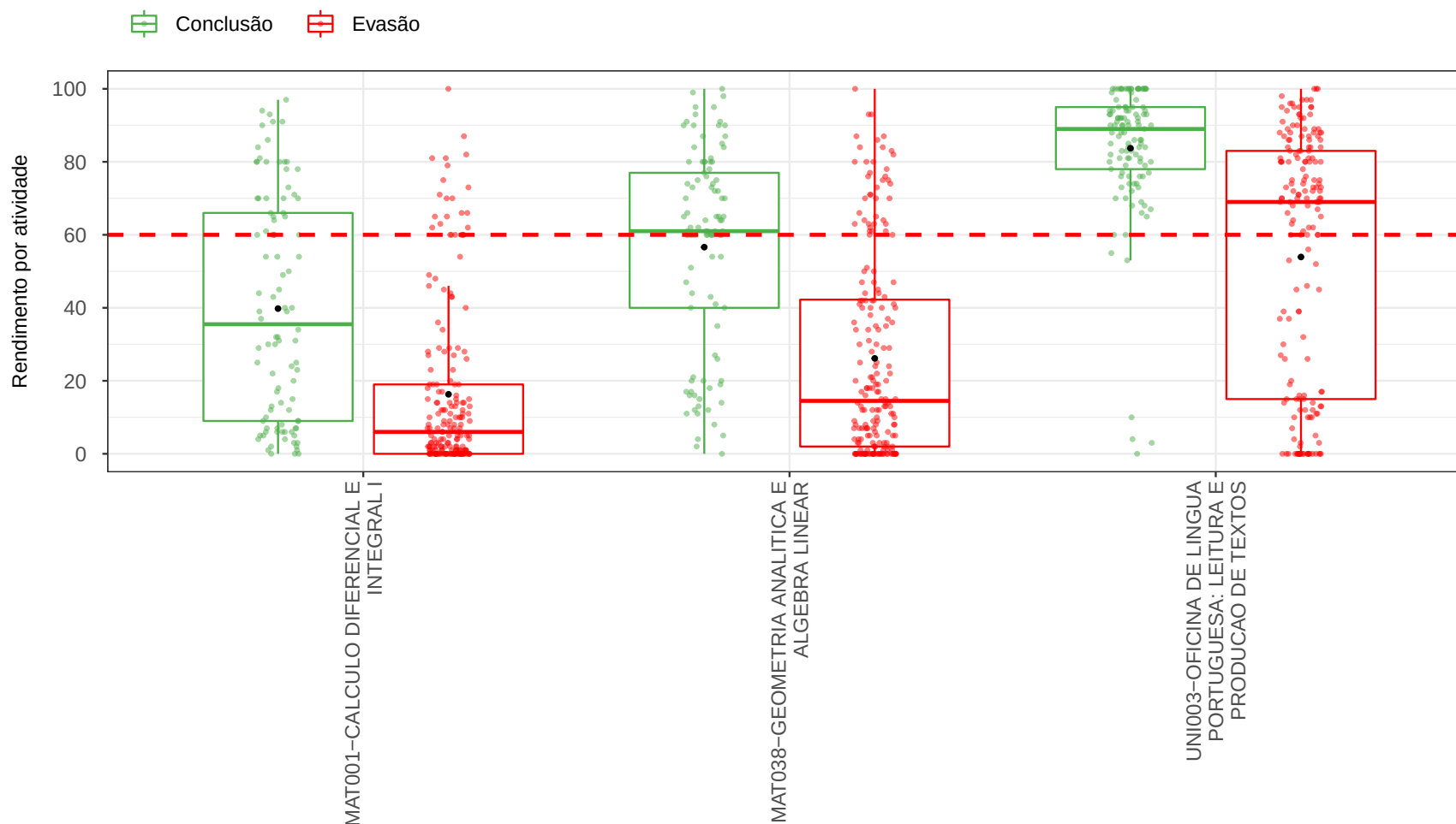
Figura 14: Rendimento por atividade acadêmica curricular, de acordo com a situação do estudante no curso de Estatística, modalidade Bacharelado. Os valores do rendimento dos estudantes são representados como pontos da mesma coloração do gráfico. A média é indicada pelo ponto de cor preta e a mediana é a linha horizontal dentro do boxplot.
