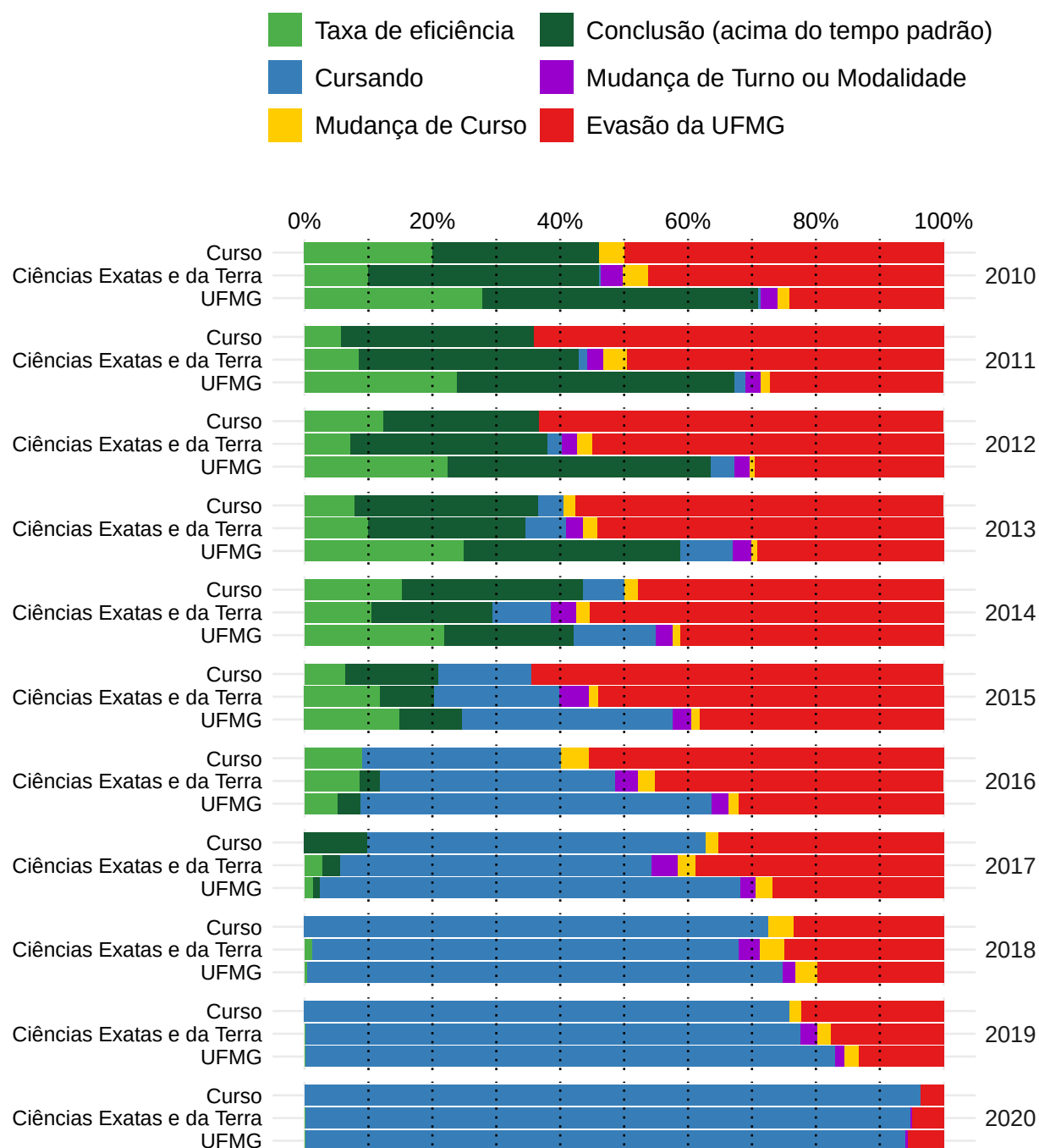
Figura 9: Situação dos estudantes do curso de Estatística (Bacharelado), após o término do período letivo de 2020/2 A taxa de eficiência refere-se à proporção de estudantes que concluíram o curso dentro do tempo padrão de integralização. Mudança de turno ou modalidade corresponde tanto à troca de diurno para noturno, e vice-versa, quanto a alteração entre as modalidades bacharelado e licenciatura. Mudança de curso troca de curso dentro da UFMG, por meio de reopção, no âmbito das vagas remanescentes (exceto casos de mudança de turno ou modalidade). Evasão da UFMG equivale ao desligamento ou evasão da UFMG sem a conclusão de curso de graduação.
