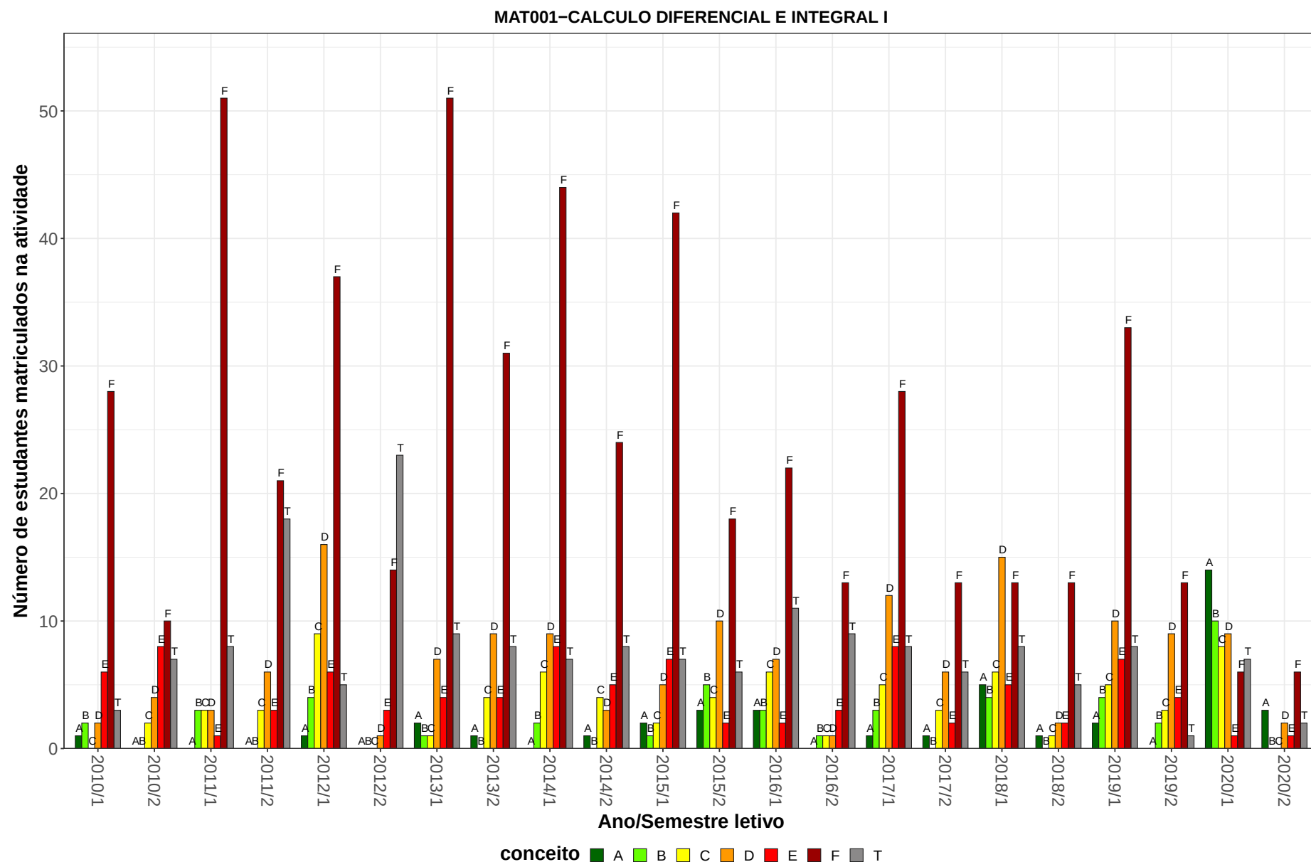
Figura 6: Conceitos obtidos pelos estudantes matriculados no curso de Estatística, modalidade Bacharelado, no período de 2010/1 a 2020/2 na atividade MAT001-CALCULO DIFERENCIAL E INTEGRAL I.
