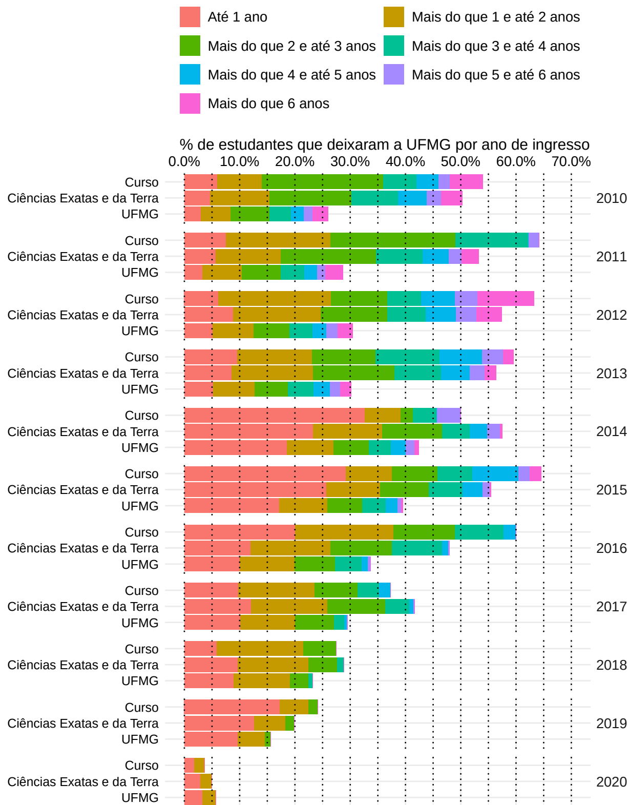
Figura 11: Taxa de Evasão Anual do curso de Estatística, modalidade Bacharelado.
