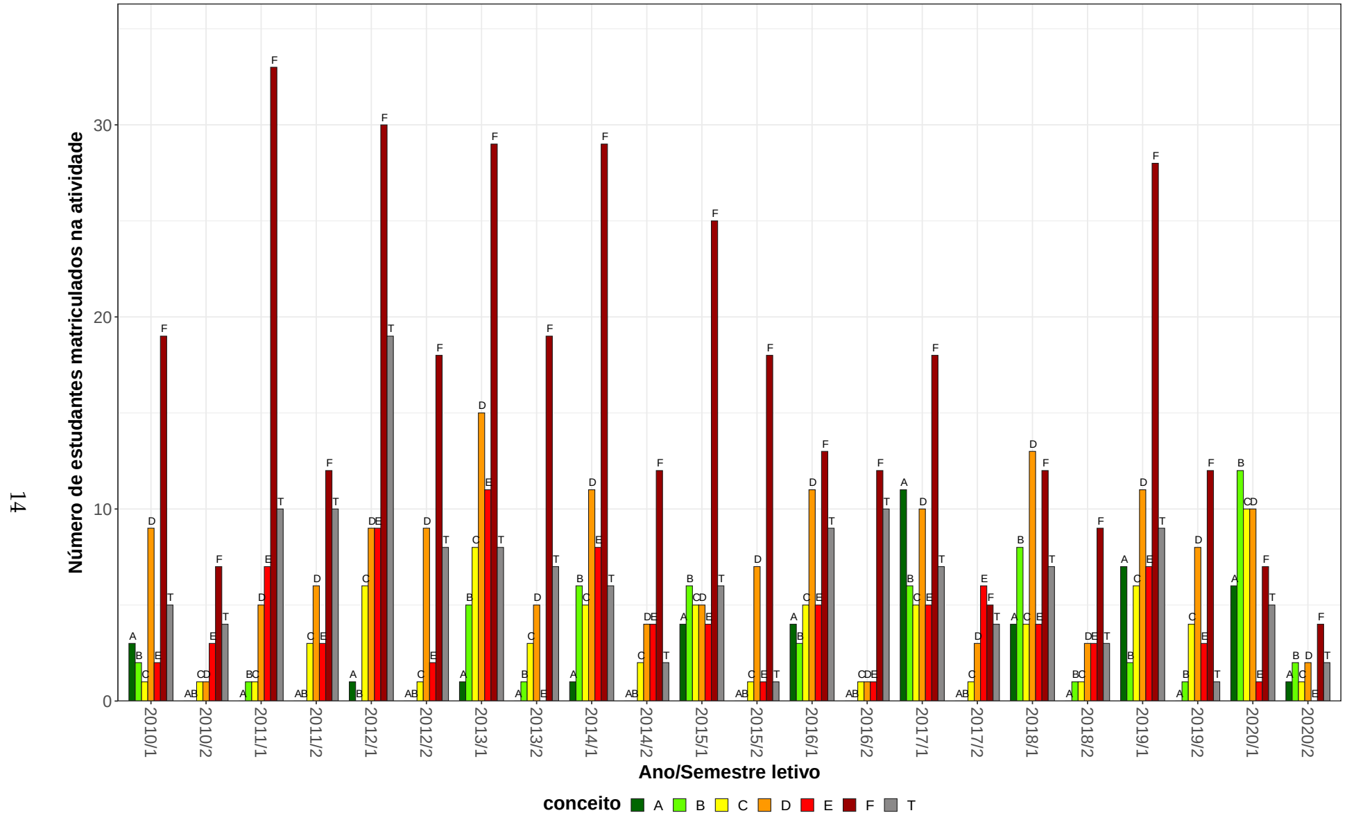
Figura 7: Conceitos obtidos pelos estudantes matriculados no curso de Estatística, modalidade Bacharelado, no período de 2010/1 a 2020/2 na atividade MAT038-GEOMETRIA ANALITICA E ALGEBRA LINEAR.
