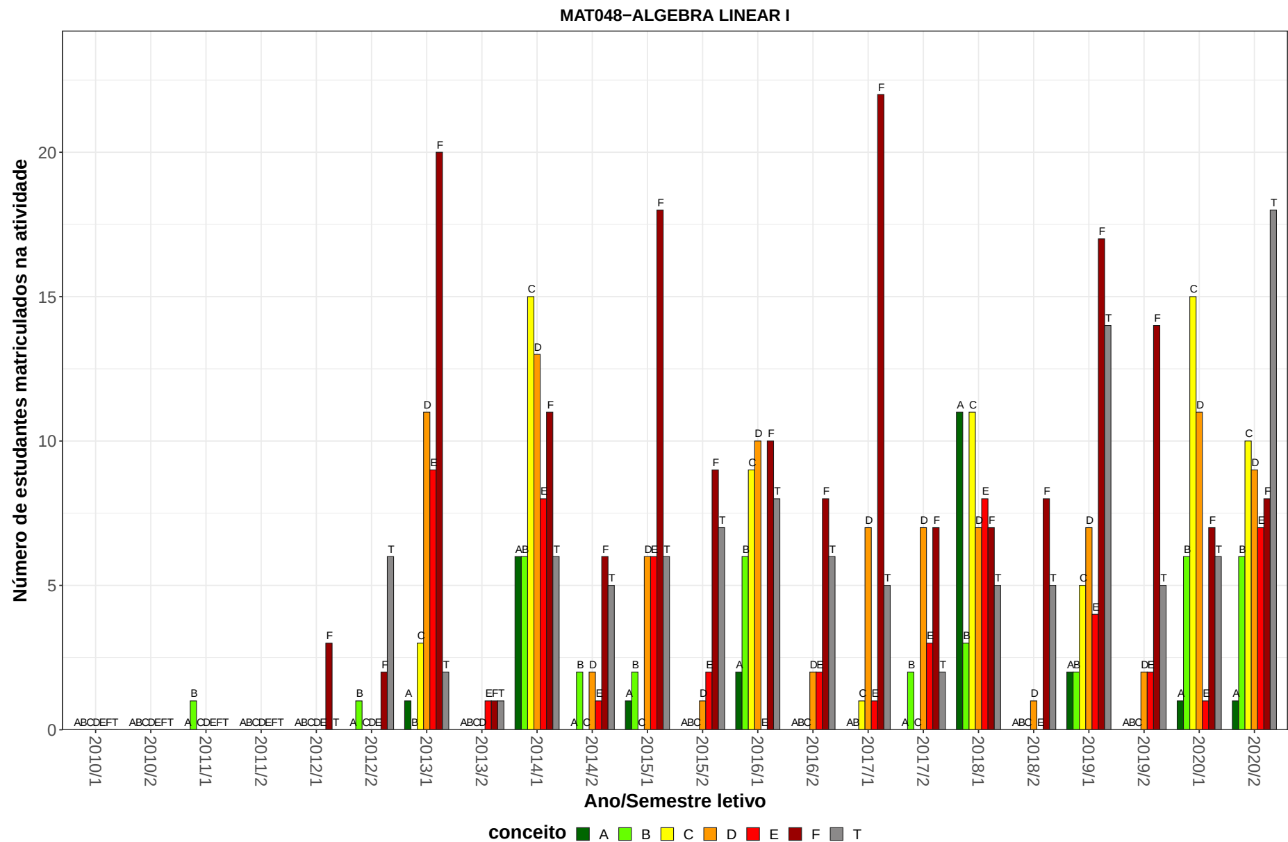
Figura 5: Conceitos obtidos pelos estudantes matriculados no curso de Estatística, modalidade Bacharelado, no período de 2010/1 a 2020/2 na atividade MAT048-ALGEBRA LINEAR I.
