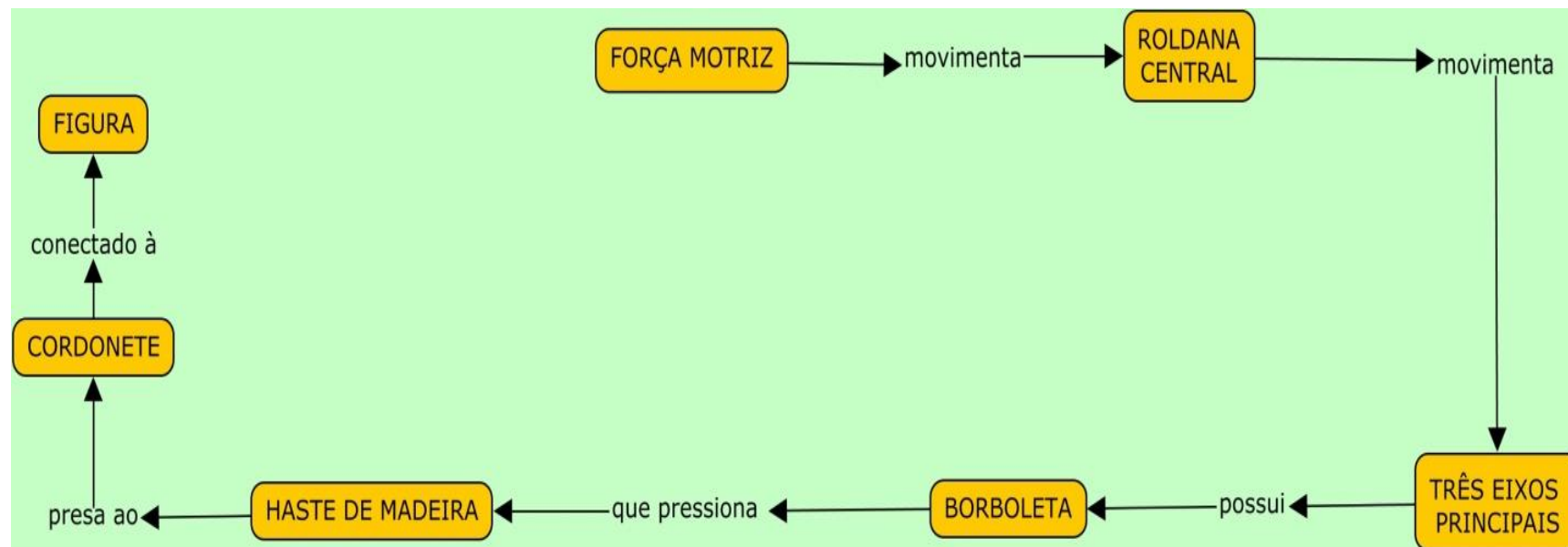
Diagrama da maquinaria do presépio
