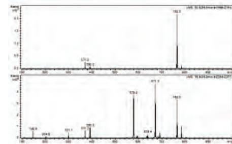
Espectro de massas para identificação das substâncias
