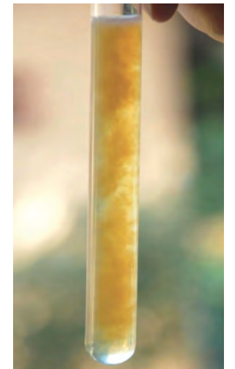
Formação do precipitado
