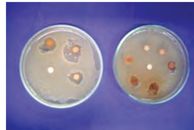
Teste in vitro : o disco é embebido em solução com extrato-seco da planta. O halo limpo ao seu redor revela a bioatividade.
